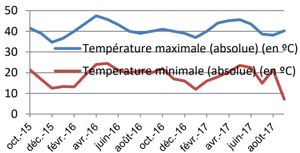
Graphique 6.2 : Evolution des températures minimales et maximales enregistrées par la station de Dori
