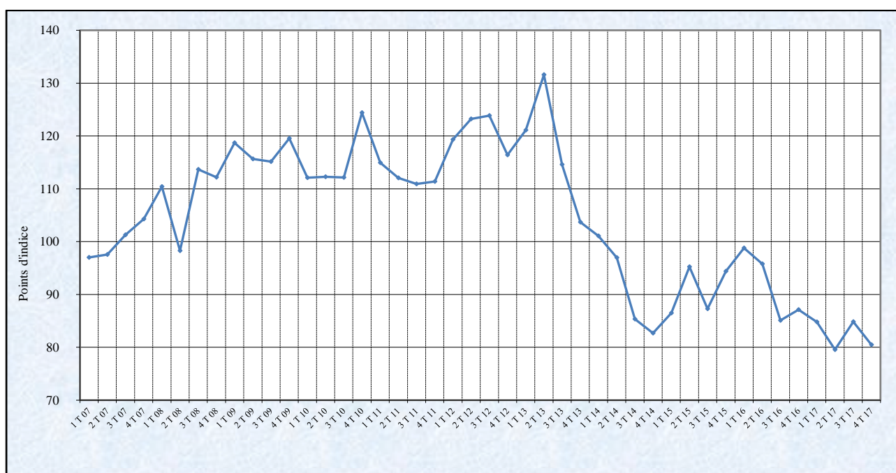
Figure 07 : Evolution trimestrielle de l'indice de Paasche des prix à l'importation depuis 2007
