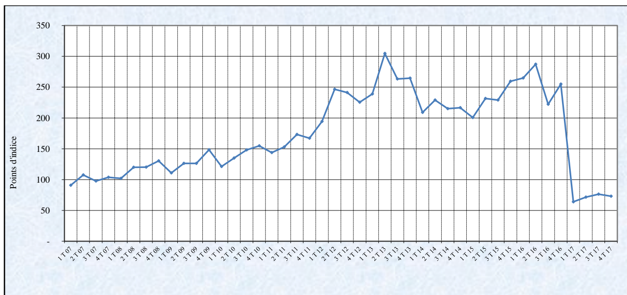
Figure 09 : Evolution trimestrielle des indices des valeurs totales à l'importation depuis 2007
