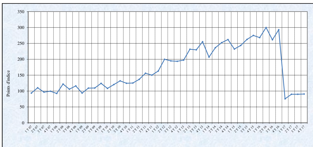
Figure 08 : Evolution trimestrielle de l'indice de Laspeyres des quantités (ILQ) à l'importation depuis 2007
